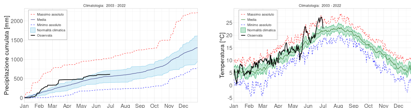
Figura 11: Andamento rispetto alla climatologia
