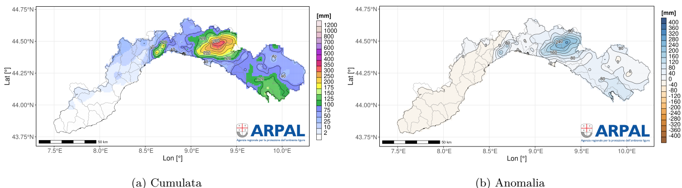
Figura 1: Precipitazione mensile
