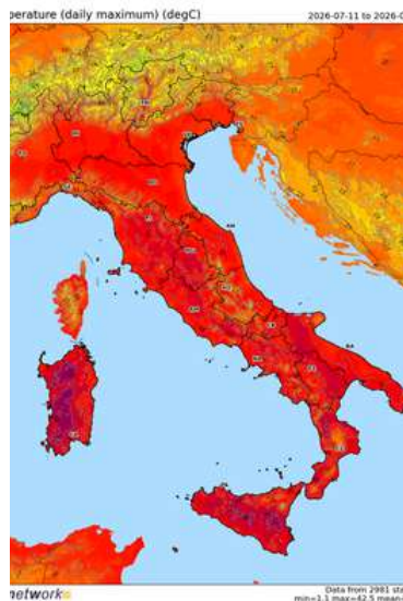
Fig. 3 le mappe Meteonetwork del 15 luglio per l'Italia (a) e la Liguria per la Temperatura massima giornaliera (b)
