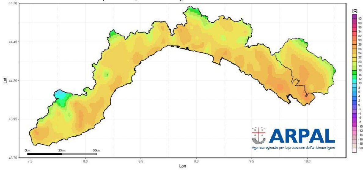
Dati di temperatura interpolati con metodo geostatistico riferiti al 03/06/2021 16:00 locali
