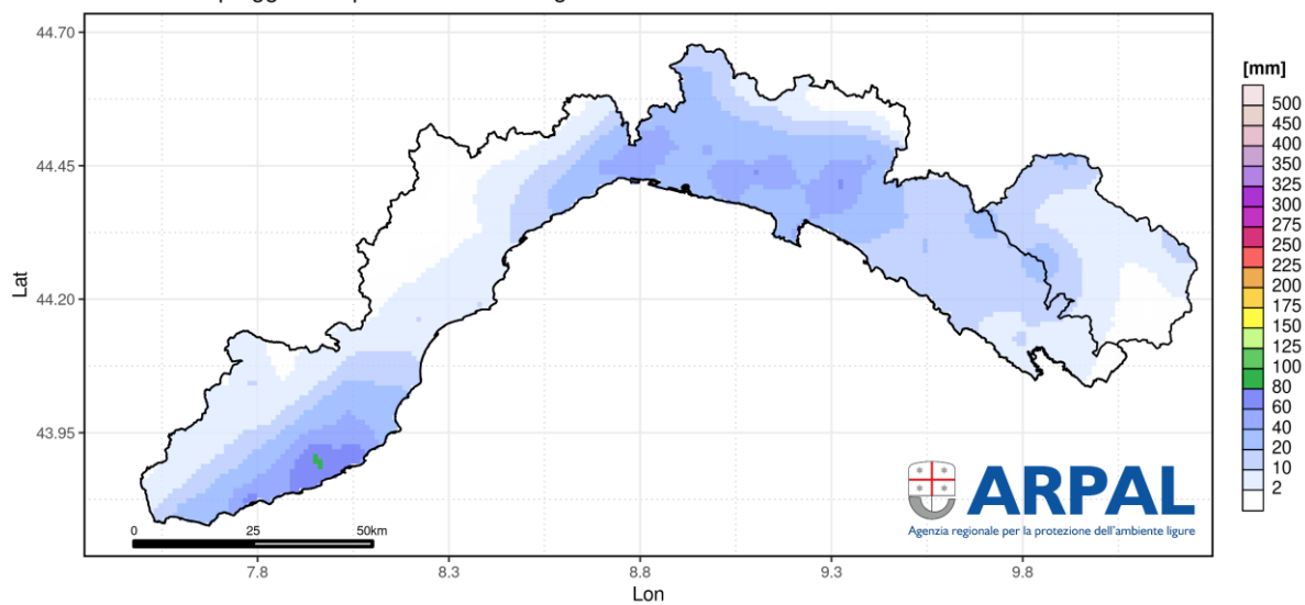
Dati di pioggia interpolati con metodo geostatistico su 24 ore riferiti al 22/12/2022 00:00 locali
