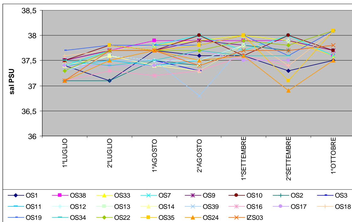
Figura 3.3 - Andamenti temporali della salinità.
