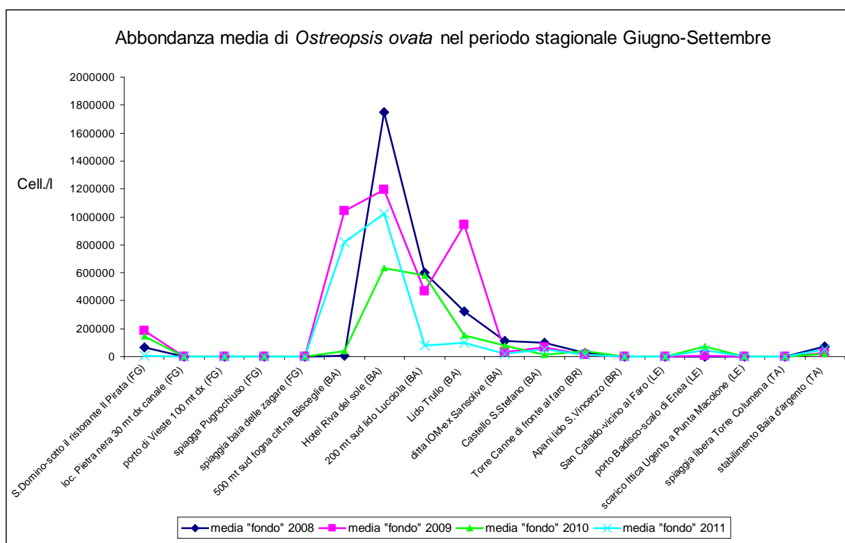
Figura 10.2 - Abbondanza media di Ostreopsis ovata nel periodo stagionale Giugno-Settembre.
