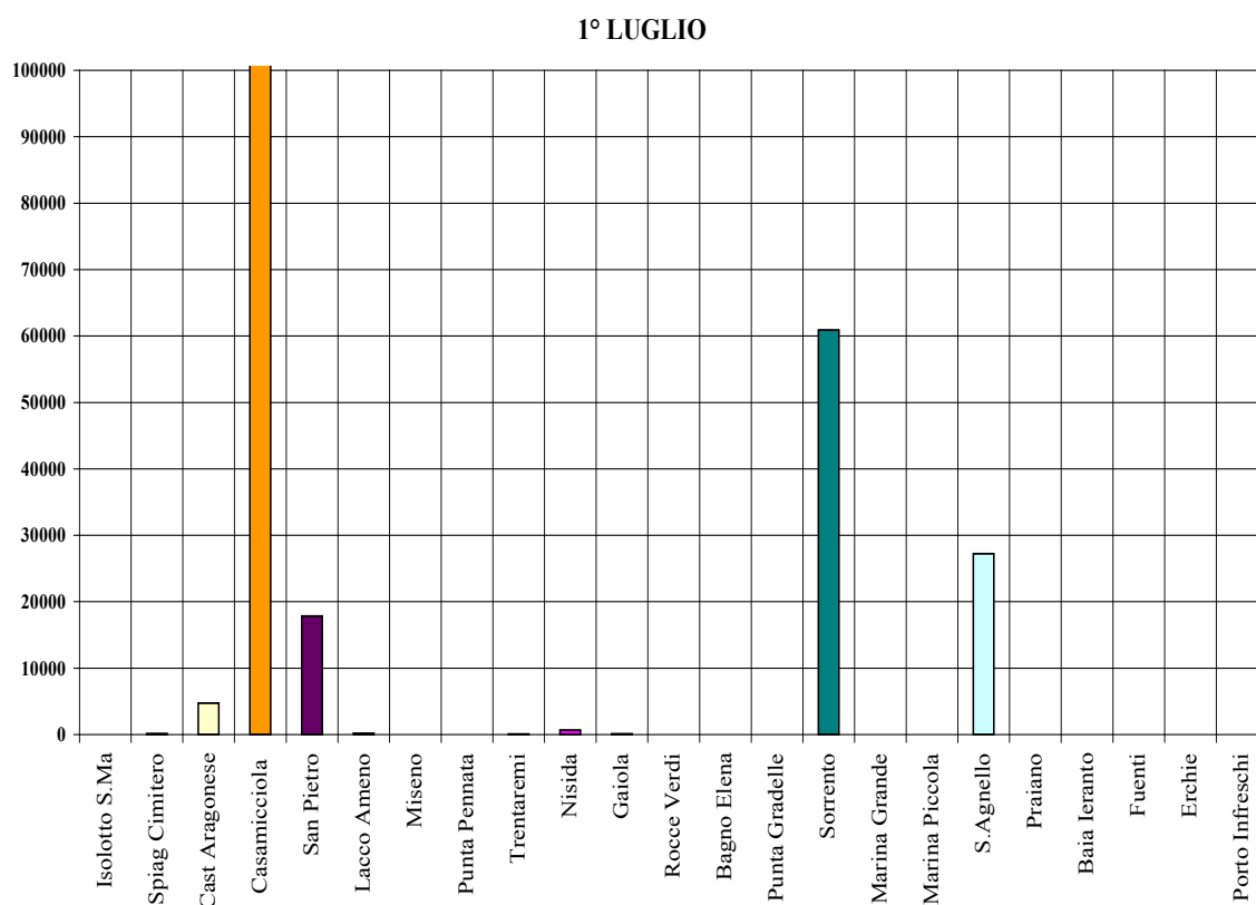
Figura 3.5 -Andamento temporale delle fioriture: 1° campagna Luglio.
