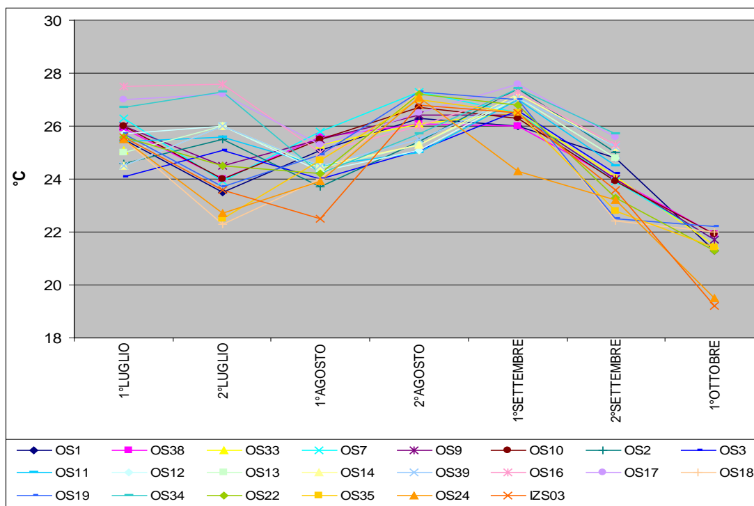
Figura 3.4 - Andamenti temporali della temperatura.
