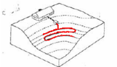
Figura 9: subirrigazione a serpentina
